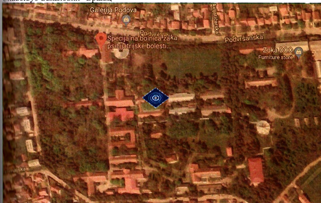
Слика 17. Сателитски снимак Специјалне болнице за психијатријске болести “Др Славољуб Бакаловић” Вршац
