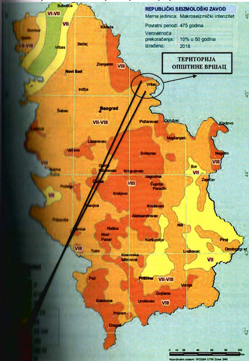
Слика 9. Карта Сеизмског хазарда Републике Србије
