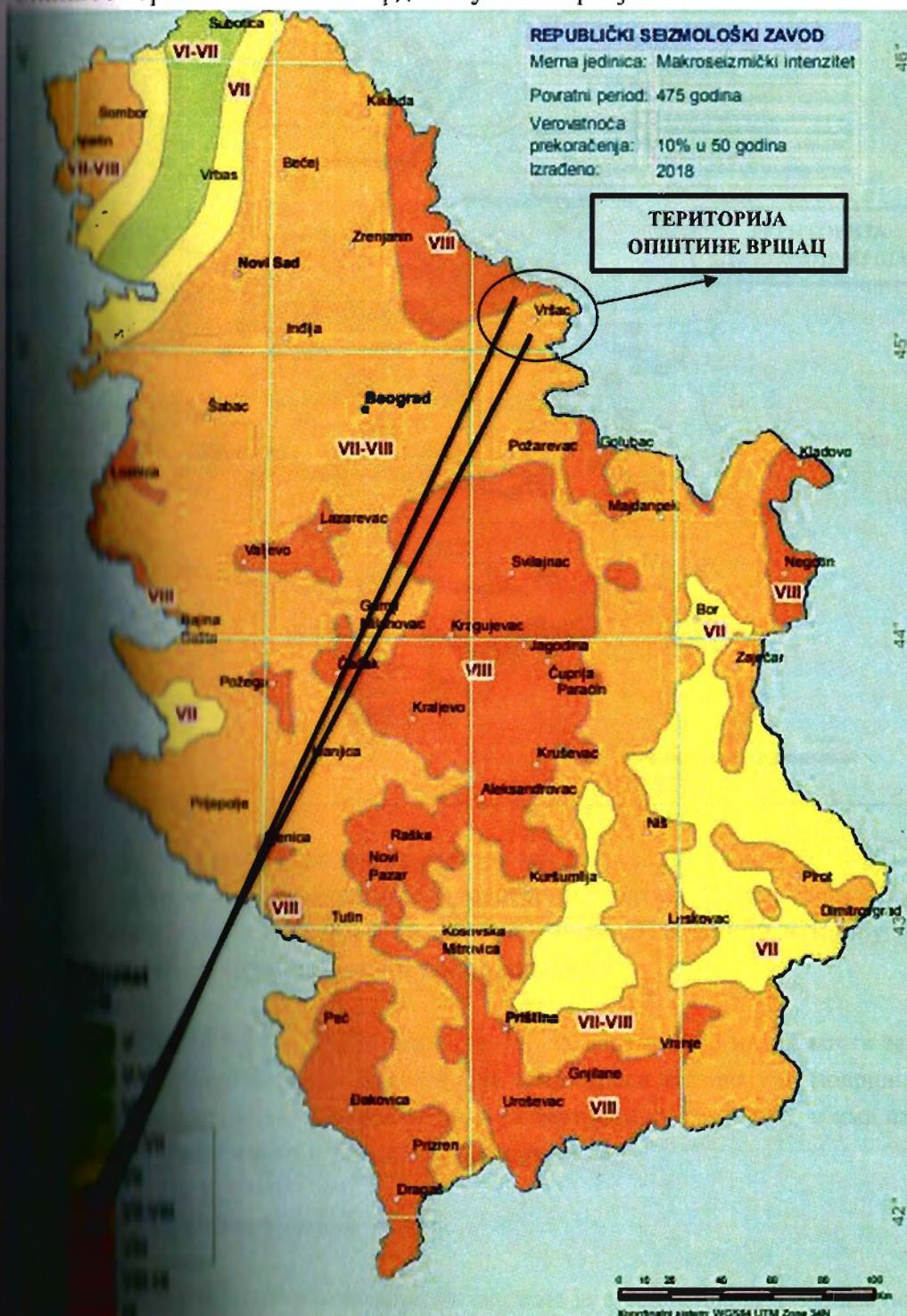
Слика 9. Карта Сеизмичког хазарда Републике Србије
