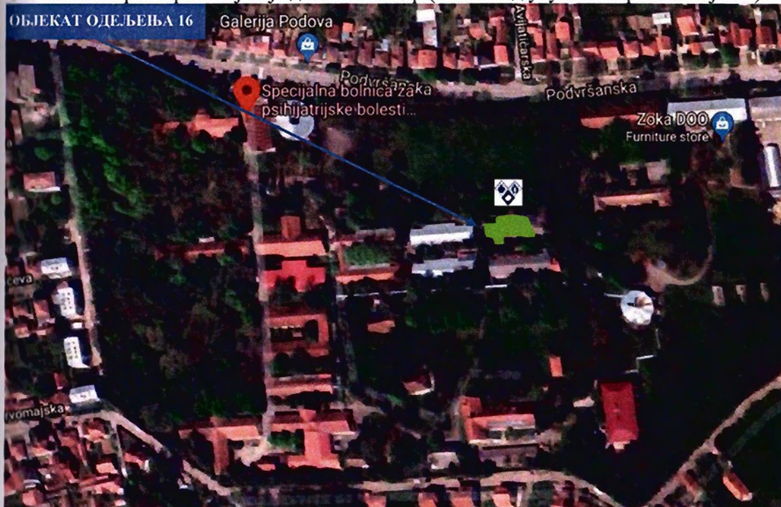
Слика 21. Простор на којем је деловао пожар ( 440 \text{ m}^2 од укупне површине објекта)
