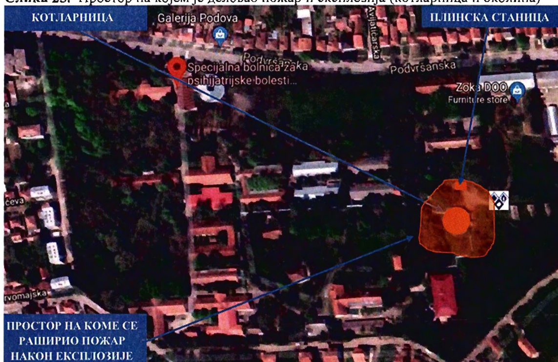
Слика 25. Простор на којем је деловао пожар и експлозија (котларница и околина)
