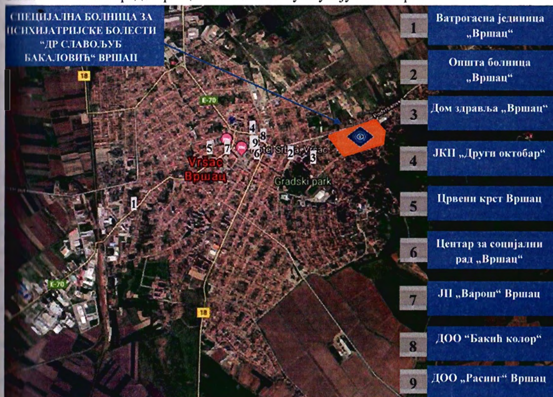
Слика 18. Снаге града Вршца за ангажовње у случају земљотреса
