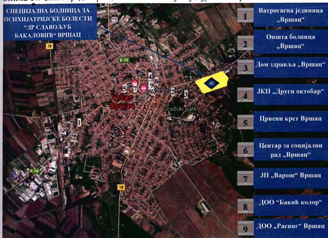
Слика 14. Снаге града Вршца за ангажовње у случају земљотреса
